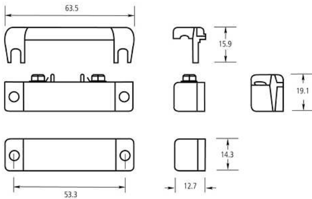
Mitat
